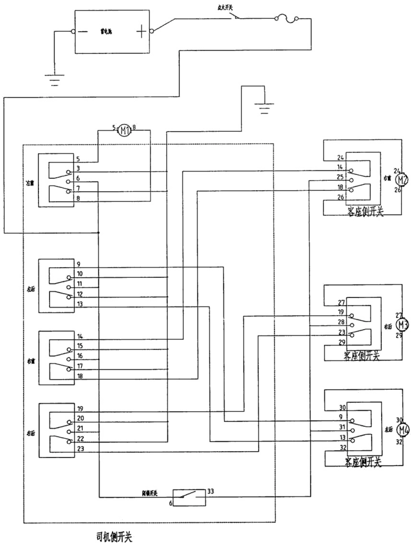
T系列电动玻璃升降器接线原理图
